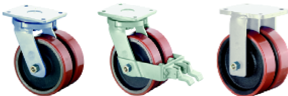
Schwerlast-Doppel-Lenkrollen Heavy-duty-double-castors
