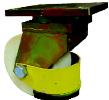
Schwerlastrollen mit Fußschutz Heavy duty castors with foot protection
