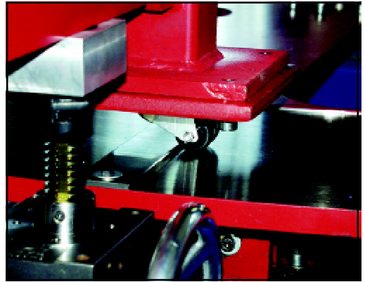
Prüfstand gemäß Europa-Norm
